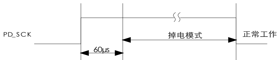
图4 掉电控制
