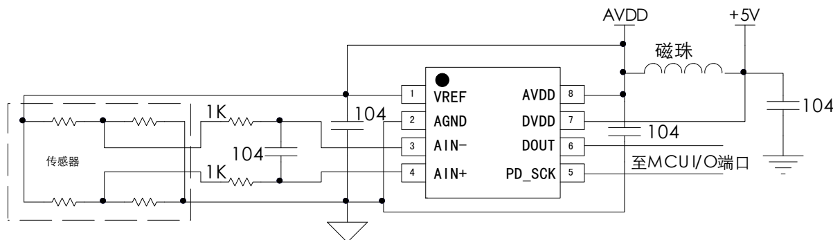
图 1 典型应用
